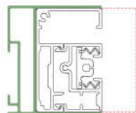
coulisses 38 / guía 38
