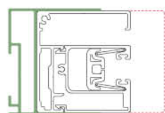
coulisses 56 / guía 56
